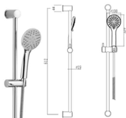
DIANA O100-Neu Handbrause 3S 3-fach verstellbare Handbrause, Ø 100 mm, mit Easy Clean Noppen, zertifiziert nach KTW, verchromt, (DI452023500)
