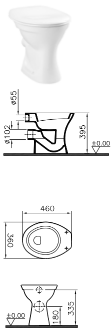
DIANA O100 Flachspül-Stand-WC** mit waagrechtm Abgang, Ausladung 460 mm, (DI000605001)
