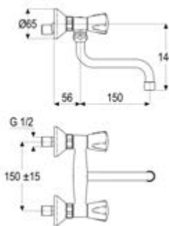
DIANA O100 2-Griff Spültisch-Wandarmatur Schwenkauslauf 150 mm, G 1/2" verchromt, (DI407763500)
