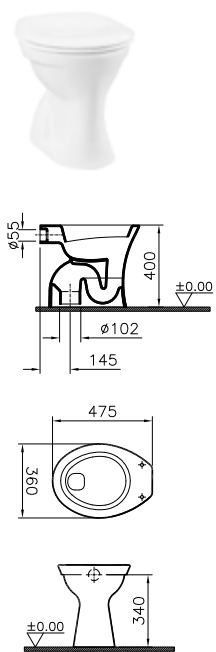
DIANA O100 Flachspül-Stand-WC** mit senkrechtem Abgang, Ausladung 475 mm, (DI000606001)
