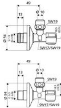
DIANA Eckventil 1/2" mit Schubrosette, 1/2", verchromt,
