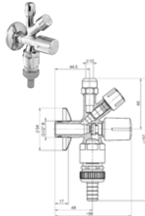
DIANA O100 Kombi-Eckventil mit selbstdichtendem Anschlussge- winde, DVGW geprüft, mit Rückfluss- verhinderer, Rohrbelüfner, Rosette und Schlauchverschraubung, poliert verchromt, (DI407955500)
