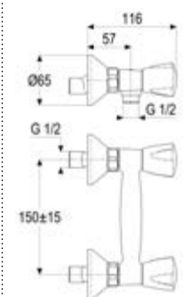
DIANA O100 Brausearmatur ohne Brausegarnitur, verchromt, (DI407301500)
