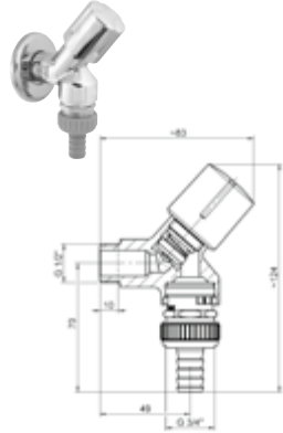
DIANA O100 Geräteschrägsitzventil mit Rückflussverhinderer, Rohrbe- löfner und Schlauchverschraubung, poliert verchromt, DVGW geprüft, (DI407943500)
