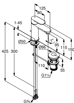
DIANA O200 Waschtischmischer 100
