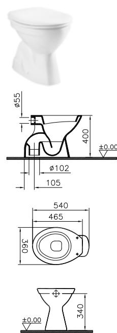
DIANA O100 Tiefspül-Stand-WC** mit senkrechtem Abgang, Ausladung 465/ 540 mm, (DI000603001)
