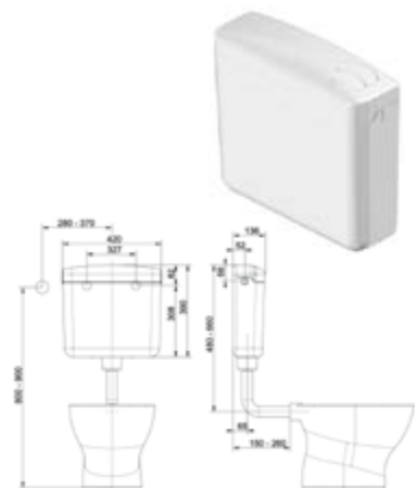
DIANA O200 Spülkasten 6–9 l mit wassersparender 2-Mengen-Technik, Spülmenge groß: von 6 l auf 9 l umstellbar, Spülmenge klein: 3 l, Weiß, (DI040500001)
