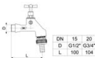
DIANA O100 Auslaufventil Oberteil mit Knebelgriff, DVGW zugelassen, mit Belüfter und Rückflussverhinderer, mit Schlauchverschraubung
