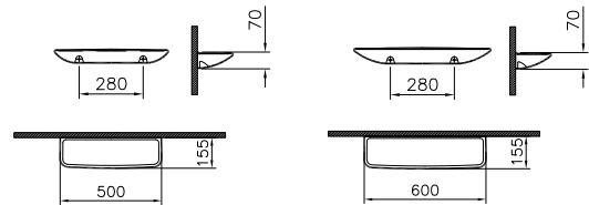
DIANA O100 Aluminium Einlegerost
