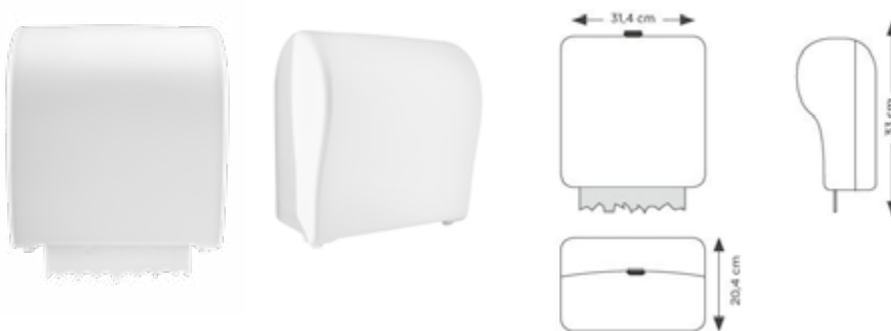
DIANA O100-Neu Rollenpapierspender für Papierhandtuchrollen mit Autocut, ABS-Kunststoff, mit Schloss, Weiß, (DI645010502)
