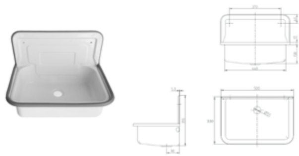
DIANA O100 Stahl Ausgussbecken
