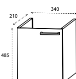
DIANA O100 WT-Unterschrank zu DIANA S100 Handwaschbecken mit 1 Tür, B 340, H 485, T 210 mm,
