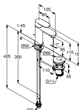
DIANA O200 Waschtischmischer 100 Niederdruck
