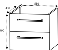
DIANA O100 WT-Unterschrank zu DIANA M100 Möbelwaschtischen bestehend aus 1 Metallauszug mit Einzugsdämpfung und Siphonausschnitt, 1 Metallauszug mit Einzugsdämpfung und Reling, H 490, T 430 mm,
