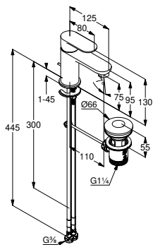
DIANA O200 Waschtischmischer 75
