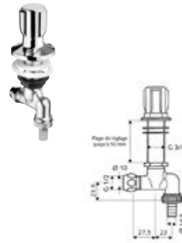
DIANA Spültischventil ohne Rohrbelüfter mit Rückflussverhinderer, und Schlauchverschraubung, Verstellbereich 1-50 mm, Dimension DN 15 x 10 mm G 1/2 AG, verchromt, (DI407971500)
