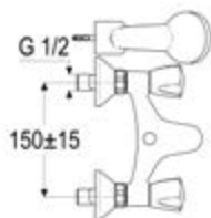
DIANA O100 Wannenarmatur eigensicher mit Brausegarnitur, Schlauch 125 cm, Wandbrausehalter, verchromt, (DI407403500)
