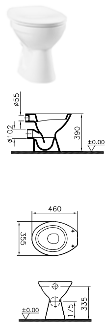
DIANA O100 Tiefspül-Stand-WC** mit waagrechtm Abgang, Ausladung 460 mm, (DI000602001)
