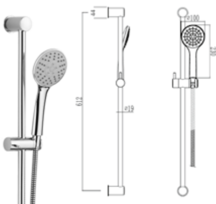
DIANA O100-Neu Brauseset 1S Brausestange 600 mm, Handbrause 1S, Schlauch 1600 mm, verchromt, zertifiziert nach KTW, (DI452321500)
