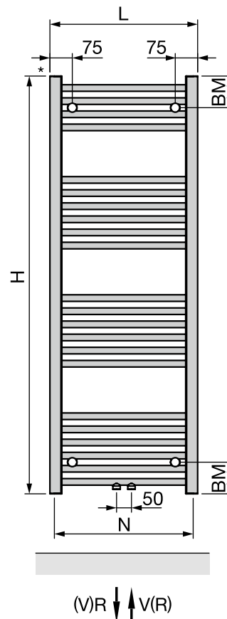
DIANA O100 Badheizkörper Vorderansicht
