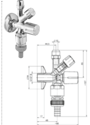
DIANA O100 Kombi-Eckventil DVGW geprüft, mit Rückflussverhinde- rer, Rohrbelüfner, Rosette und Schlauch- verschraubung, poliert verchromt, (DI407954500)
