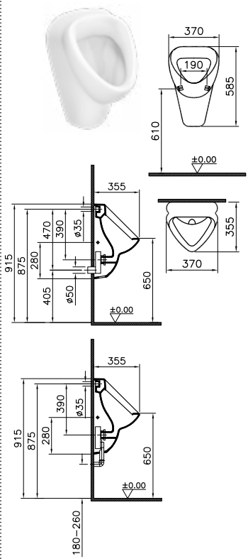
DIANA O100 Urinal** Zulauf von hinten, mit Spülrand, Abgang universal, (DI000801001)
