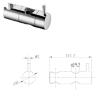
DIANA O100-Neu Ersatzgleiter für Ø 19 mm, mit Stifthebel, verchromt, (DI452603500)
