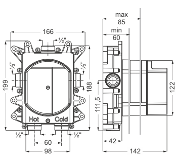
DIANA L Universal Einbaubox für Wannen-/ Brause- und Thermostat-Endmontagesets, 3 Abgänge rechts/ links/oben getrennt ansteuerbar, 2 Zulaufe unten verwechslungssicher markiert, Spül- und Abdruckvorrichtung, Anschlussmaße 1/2", Flies-Dichtmanschette, 2 Blindstopfen für nicht benötigte Abgänge, schallentkoppelte Montage, Einbautiefe 60 mm – 85 mm, (DI406510) 160,- €
