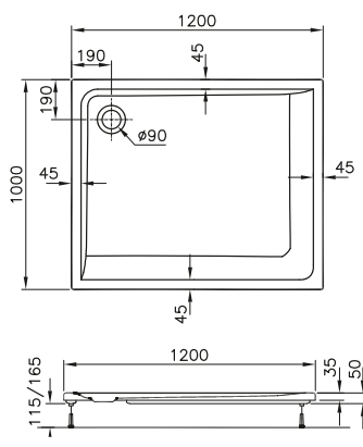
DIANA M100 Acryl-Rechteck-Duschwanne Weiß, 1200 x 1000 mm, Tiefe 35 mm, Ablaufloch 90 mm, (DI225024001) 637,- €
