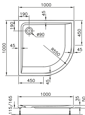
DIANA M100 Acryl-Viertelkreis-Duschwanne Weiß, 1000 x 1000 mm, Tiefe 35 mm, Ablaufloch 90 mm, (DI225054001) 641,- €
