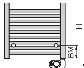
Detailzeichnung elektrisch
