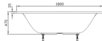
DIANA M100 Acryl-Duo-Einbauwanne Weiß, 1800 x 800 mm, Nutzinhalt ca. 264 Liter, (DI205014001) 692,- €
