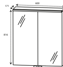
DIANA O100 Spiegelschrank inkl. 2 Doppelspiegeltüren, 2 Glasfach- böden, 1 Gesimsboden mit LED- Beleuchtung und 15,0 Watt Converter, 1 Schalter-Steckdosen- Element eingebaut H 816, T 171 mm,
