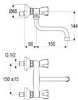
DIANA O100 2-Griff Spültisch-Wandarmatur Schwenkauslauf 150 mm, G 1/2" verchromt, (DI407763500) 137,- €
