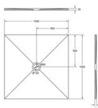
DIANA L300-Neu Mineralguss Duschwanne 1000 x 1000 mm, Tiefe 25 mm, Ablaufloch 90 mm, Oberfläche strukturiert, Weiß, (DI226414001) 713,- € Grau, (DI226414052) 713,- € Anthrazit, (DI226414030) 713,- €
