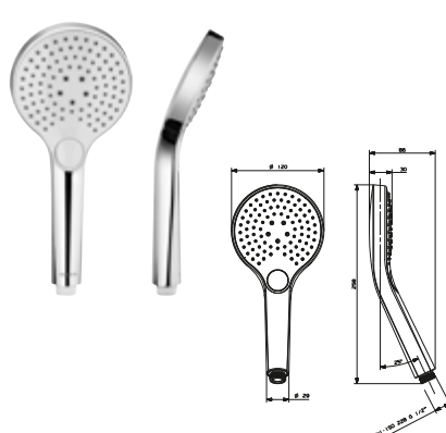
DIANA M100 Eco Handbrause 120 mm 3S Brauseregen, Weichstrahl-Gemischter Strahl, mit Drückknopf, Kalk Easy-Clean, (DI455103500) 76,90 €
