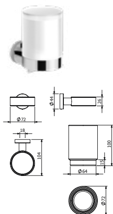
DIANA M200-Neu Wand-Seifenspender Bedienung von unten, mit Stülpbehälter aus Kristallglas matt, Füllmenge ca. 160 ml,
