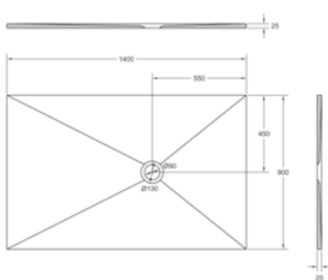
DIANA M300-Neu Mineralguss Duschwanne glatt, Weiß, 1400 x 900 mm, Tiefe 25 mm, Ablaufloch 90 mm, (DI226343001) 826,- €
