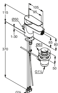
Auslaufhöhe 65 mm, Ausladung 105 mm, Einlochmontage, verstellbarer S-Pointer M24 PCA Strahlregler, Keramik-Kartusche mit Heißwasser- begrenzung, Schnell-Montagesystem, flexible Anschlüsse G 3/8, verchromt, (DI1401240500) 265,- €
