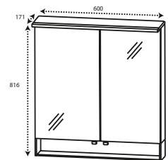
DIANA O100 Spiegelschrank inkl. 2 Doppelspiegeltüren, 2 Glasfach- böden, 1 offenes Fach, 1 Gesims- boden mit LED-Beleuchtung und 15,0 Watt Converter, Türhöhe in 636 mm, 1 Schalter-Steckdosen- Element eingebaut H 816, T 171 mm,
