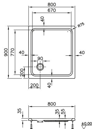
DIANA S100 Acryl-Rechteck-Duschwanne Weiß, 900 x 800 mm, Tiefe 35 mm, Ablaufloch 90 mm, (DI224202001) 397,- €
