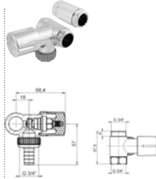
DIANA O100 Nebenanschlussventil für Wandbatterien, mit Rückflussver- hinderer und Schlauchverschraubung, poliert verchromt, mit Distanzstück zur Montage von Wandbatterien, Anschluss rechts, (DI407944500) 65,10 €
