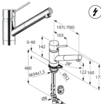
DIANA K200 Spültisch-Einhandmischer, Niederdruck mit schwenkbarem und herausziehbarem Auslauf, für drucklose Speicher, verchromt, (DI427205500) 436,- €
