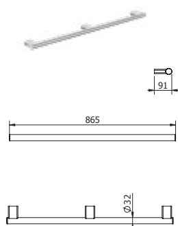
DIANA C100 Haltegriff verchromt, gerade, mit Mittelkonsole, 865 mm, (DI617014500) 230,- €
