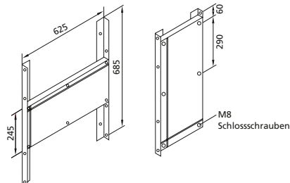
DIANA BS+ Montageplatte Universal Schichtholzplatte 625 x 245 mm, Plattenstärke 30 mm, mit 2 Befestigungswinkeln, 685 mm lang, (DI061910) 85,80 €
