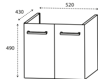
DIANA O100 WT-Unterschrank für LAUFEN Pro A mit 2 Türen, H 490, T 430 mm,
