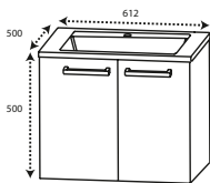
DIANA O100 Mineralguss- Waschtisch-Unterschrank SET mit 2 Türen inkl. Mineralguss Waschtisch mit Diana CLOU Ab- und Überlaufsystem in Weiß H 500, T 500 mm,
