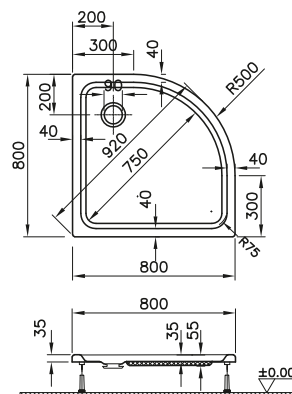
DIANA S100 Acryl-Viertelkreis-Duschwanne Weiß, 800 x 800 mm, Tiefe 35 mm, Ablaufloch 90 mm, (DI224251001) 378,- €
