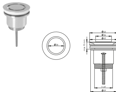
DIANA Design-Universalventil 1 1/4" x Ø 63 mm, für Becken ab Stärke 0.1 mm, Stopfen herausnehmbar, Stopfen Ø 36 mm, nicht verschließbar, Messing verchromt, (DI481028500) 60,70 €
