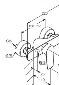
DIANA S200 Aufputz Brausemischer Durchflussmenge 28 l/min bei 3 bar, Keramik-Kartusche mit Heißwasserbegrenzung, verchromt, (DI401340500) 191,- €
