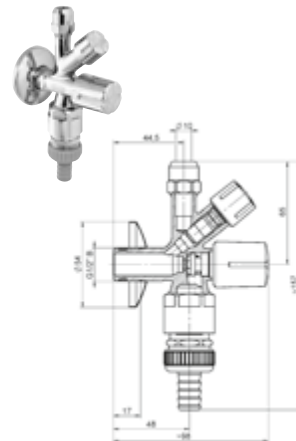
DIANA O100 Kombi-Eckventil mit selbstdichtendem Anschlussge- winde, DVGW geprüft, mit Rückfluss- verhinderer, Rohrbelüfter, Rosette und Schlauchverschraubung, poliert verchromt, (DI407955500) 61,30 €
