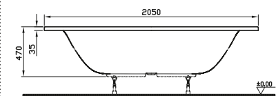
DIANA M100 Acryl-6-Eck-Einbauwanne Weiß, 2050 x 900 mm, Nutzinhalt ca. 256 Liter, (DI205064001) 1.170,- €
