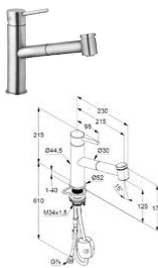
DIANA K800-Steel-Neu Spültischmischer mit Handbrause Edelstahl gebürstet, (DI423510730) 598,- €
