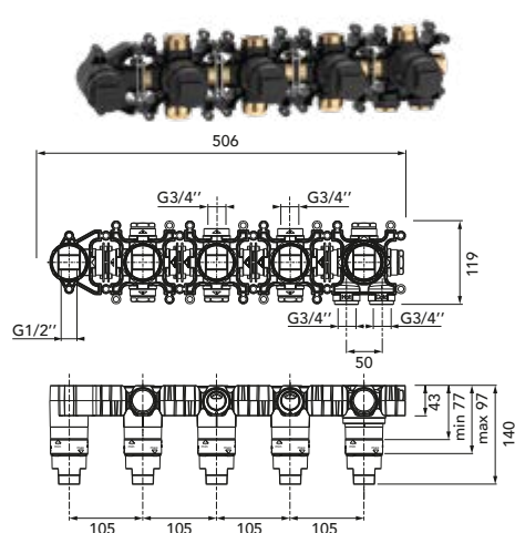
DIANA L200 Einbaukörper für Push Thermostat 3 Verbraucher (DI407613) 1.782,- €
