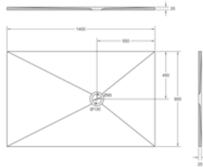
DIANA L300-Neu Mineralguss Duschwanne 1400 x 900 mm, Tiefe 25 mm, Ablaufloch 90 mm, Oberfläche strukturiert, Weiß, (DI226443001) 962,- € Grau, (DI226443052) 962,- € Anthrazit, (DI226443030) 962,- €
