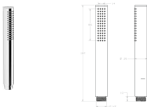
DIANA L100 Stabhandbrause Stabhandbrause aus Metall, voller Brauseregen 1-strahlig, verchromt, (DI457050500) 88,20 €
