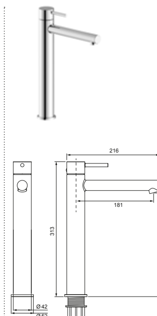
DIANA L200 Waschtischmischer XL-Size Auslaufhöhe 241 mm, Ausladung 181 mm,
