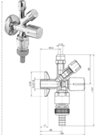
DIANA O100 Kombi-Eckventil DVGW geprüft, mit Rückflussverhinde- rer, Rohrbelüfter, Rosette und Schlauch- verschraubung, poliert verchromt, (DI407954500) 60,10 €
