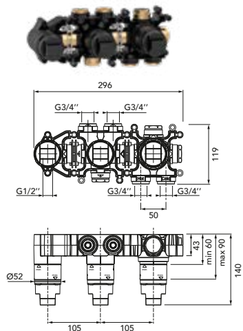
DIANA L200 Einbaukörper für Thermostat 3 Verbraucher (DI407603) 1.011,- €
