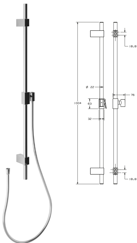
DIANA L100 Wandstange rund aus Metall 1000 mm, mit Schlauch 1600 mm, eckigem Metallschieber und eckiger Wandhalterung, verstellbar, verchromt, (DI457212500) 204,- €
