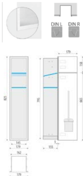
DIANA L100 WC Wand-Einbaurahmen für DIANA WC Wand-Einbauelement (DI608109) 174,- €
