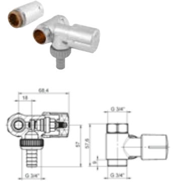
DIANA O100 Nebenanschlussventil für Wandbatterien, mit Rückflussverhinderer und Schlauch- verschraubung, poliert verchromt, mit Distanzstück zur Montage von Wandbatterien, Anschluss links, (DI407945500) 65,10 €
