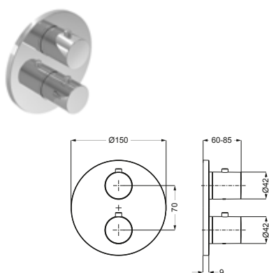
DIANA L Unterputz Thermostat
