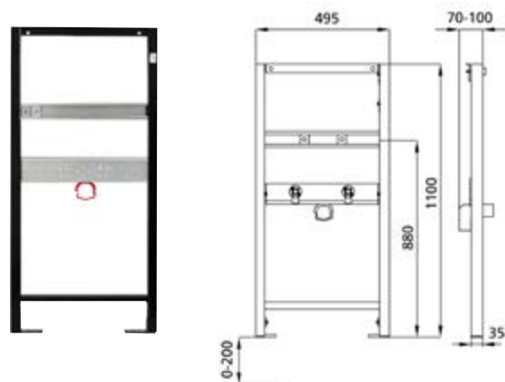
DIANA O100 Waschtisch-Leichtbauelement Bauhöhe 110 cm für Standarmatur (DI062030) 119,- €
