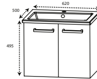
DIANA O100 Waschtischunterschrank SET mit 2 Türen inkl. Keramik-Waschtisch in Weiß mit Überlaufloch, H 495, T 500 mm,
