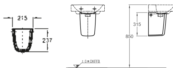
DIANA M100 Halbsäule klein für Handwaschbecken, (DI002318001) 111,- €
