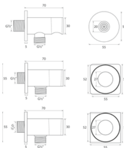
DIANA Wandanschlussbogen mit Brausehalter eigensicher, Messingausführung
