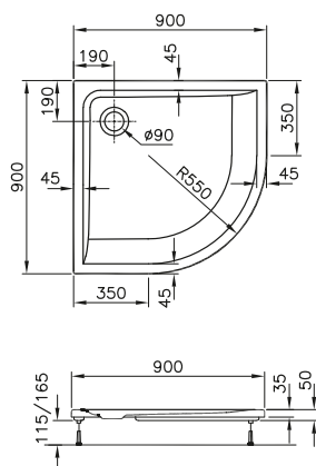
DIANA M100 Acryl-Viertelkreis-Duschwanne Weiß, 900 x 900 mm, Tiefe 35 mm, Ablaufloch 90 mm, (DI225053001) 493,- €
