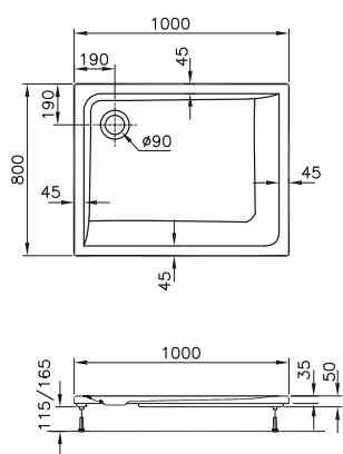
DIANA M100 Acryl-Rechteck-Duschwanne Weiß, 1000 x 800 mm, Tiefe 35 mm, Ablaufloch 90 mm, (DI225016001) 507,- €
