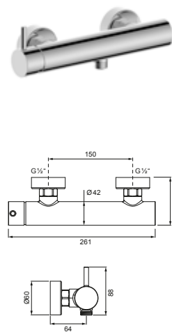
DIANA L200 Aufputz Brausemischer ohne Brausegarnitur, Brausean- schluss 1/2", SoftEmotion-Keramik- kartusche, eigensicher gegen Rückfließen, schraubbare Wandrosetten, S-Anschlüsse 1/2" / 3/4",
