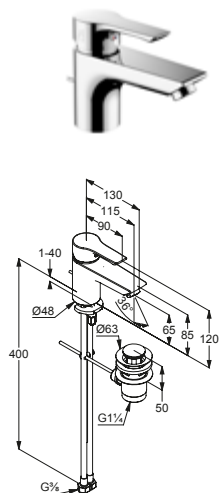
DIANA S100 Waschtischmischer Auslaufhöhe 65 mm, 1-Loch Montage, geschlossener Hebel, Keramik-Kartusche mit Heißwasserbegrenzung, Strahlregler M24, Durchflussmenge bei 3 bar 5,0 l/min, Schnell-Montagesystem, verchromt,
