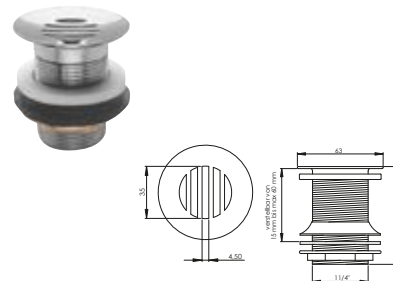
DIANA Schaftventil 1 1/4" x Ø 63 mm mit Siebeinlauf, ohne Überlaufschlitze, Schaftlänge: 70 mm, Messing verchromt, (DI481013500) 30,30 € Schwarz matt, (DI481013530) 87,- € NEU Edelstahloptik, (DI481013730) 34,- €
