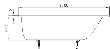
DIANA M100 Acryl-Einbauwanne Weiß, 1700 x 750 mm, Nutzinhalt ca. 264 Liter, (DI205002001) 494,- €
