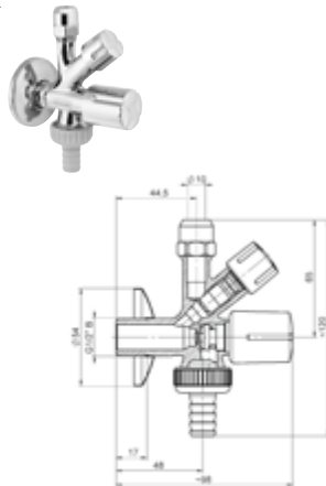
DIANA O100 Kombi-Eckventil DVGW geprüft, mit Rückfluss- verhinderer, Rosette und Schlauch- verschraubung, poliert verchromt, (DI407952500) 41,60 €
