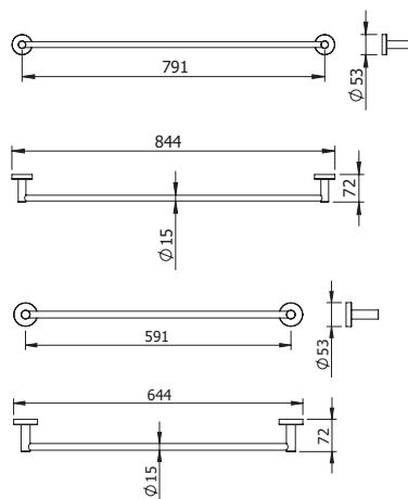
DIANA O100 Badetuchhalter verchromt, 644 mm, (DI601407500) 61,10 € 844 mm, (DI601408500) 71,10 €
