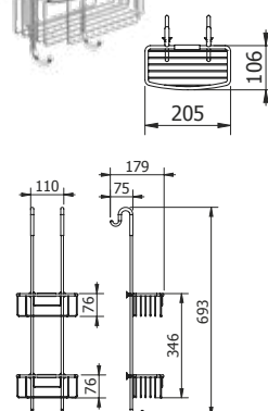
DIANA S100 Einhängeduschkorb verchromt, mit 2 tiefen Körben, Aufnahme für Wischer, ohne Wischer, (DI606571500) 253,- €
