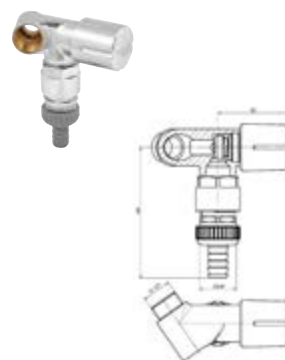
DIANA O100 Nebenanschlußventil mit Rückflussverhinderer, Rohrbelüfter und Schlauchverschraubung, poliert verchromt, DVGW geprüft, (DI407933500) 88,10 €
