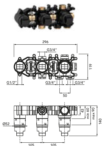
DIANA L200 Einbaukörper für Thermostat 2 Verbraucher (DI407602) 986,- €
