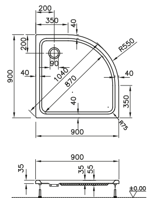
DIANA S100 Acryl-Viertelkreis-Duschwanne Weiß, 900 x 900 mm, Tiefe 35 mm, Ablaufloch 90 mm, (DI224252001) 386,- €
