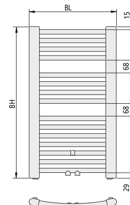
Vorderansicht
