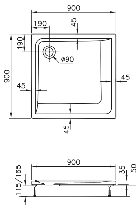
DIANA M100 Acryl-Duschwanne Weiß, 900 x 900 mm, Tiefe 35 mm, Ablaufloch 90 mm, (DI225003001) 452,- €
