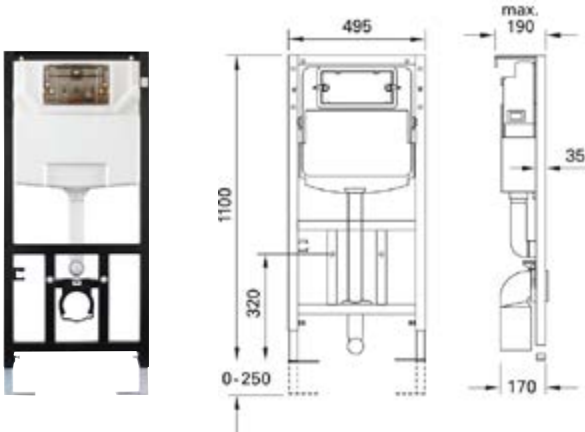
DIANA O100 WC-Leichtbau-Montageelement für WWC Bauhöhe 110 cm mit UP-Spülkasten DIANA O100 für Betätigung von vorne, für 2-Mengen-Spülung, (DI062000) 260,- €
