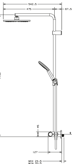
DIANA L100 Duschsystem mit Thermostat runde Kopfbrause Air-Technik 250 mm, Handbrause Air-Technik 120 mm 3S (Strahlarten: Rain, Massage, Rain und Massage) mit Brauseschlauch 1/2"x1600 mm drehbar, Rohr 22 mm, kürzbar, mit Metall- schieber und Metallwandhalterung mit Thermostat, verchromt, (DI457805500) 1.280,- €
