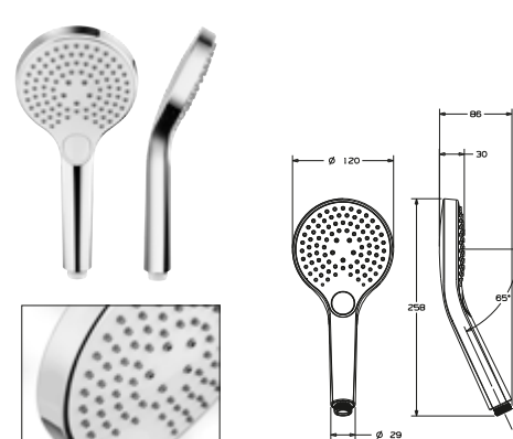
DIANA M100 Eco Handbrause 120 mm 3S mit Feinregen Feinregen-Weichstrahl-Gemischter Strahl, mit Drück- knopf, 1/2", Kalk Easy-Clean, (DI455104500) 85,60 €
