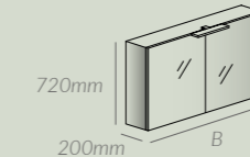
Spiegelschrank inkl. LED B 750mm LA090200* B 900mm LA090201* B 1050mm LA090202* B 1200mm LA090203*
