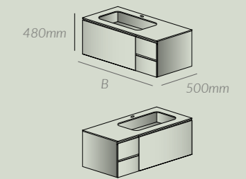
Keramikwaschtisch mit Unterschrank 1 Auszug 2 Schubladen rechts B 1050mm LA090111* B 1200mm LA090113*
